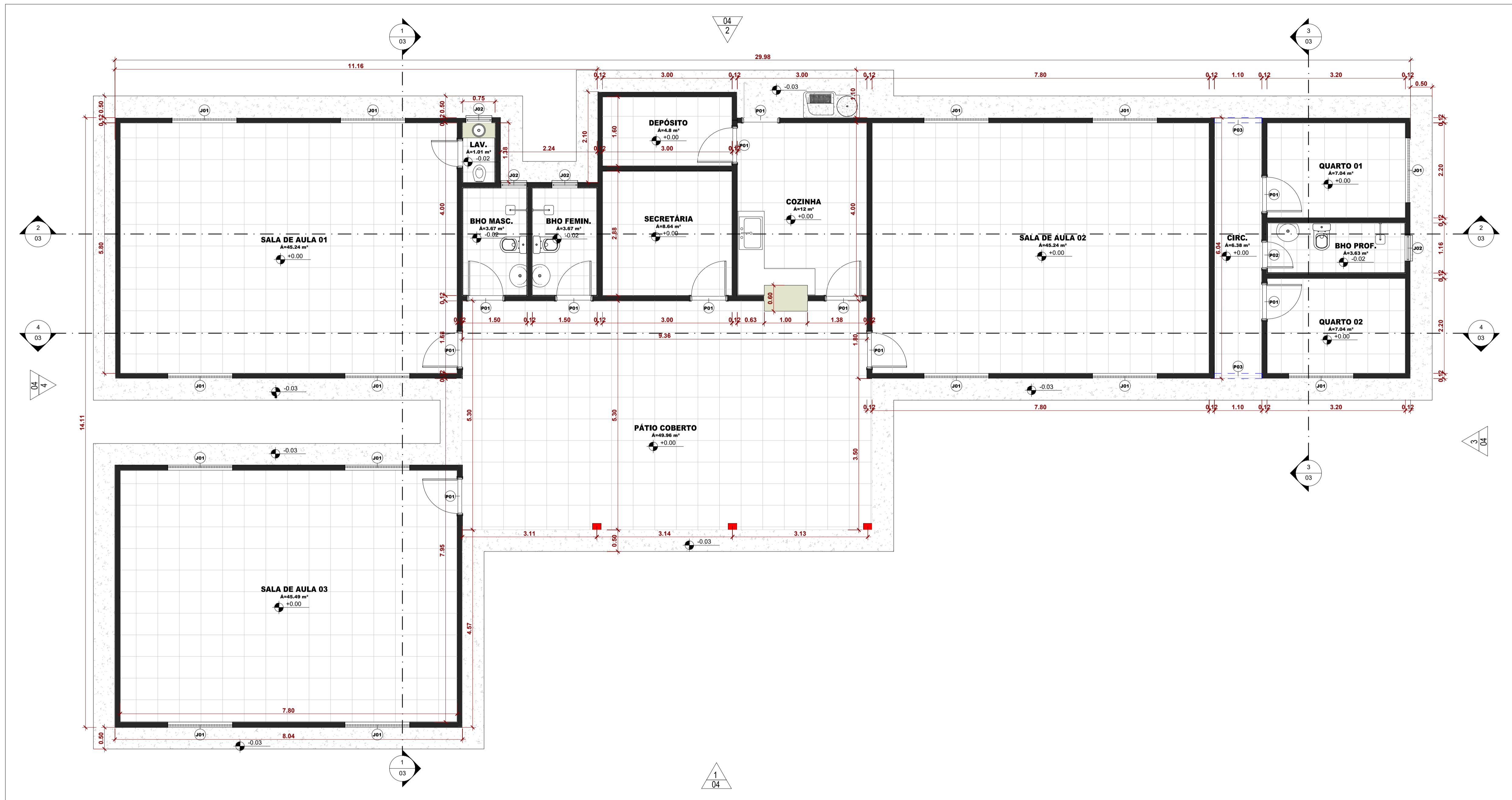
1 Planta Baixa 1 : 50
