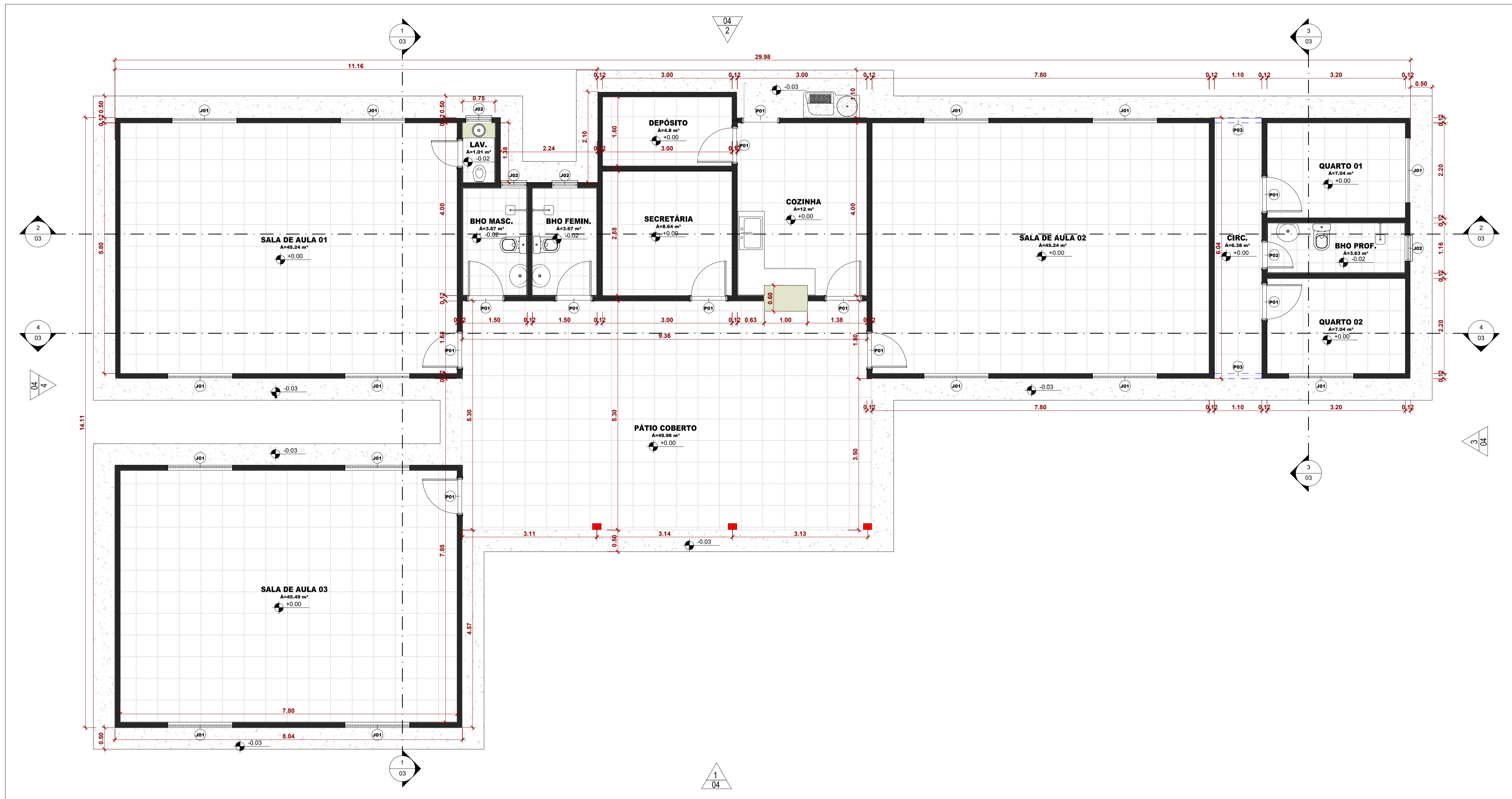
1 Planta Baixa 1 : 50
