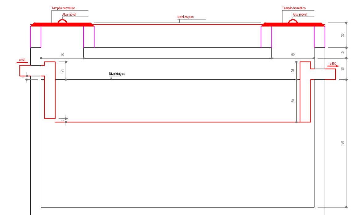
TANQUE SÉPTICO CORTE - ESC. 1:25
