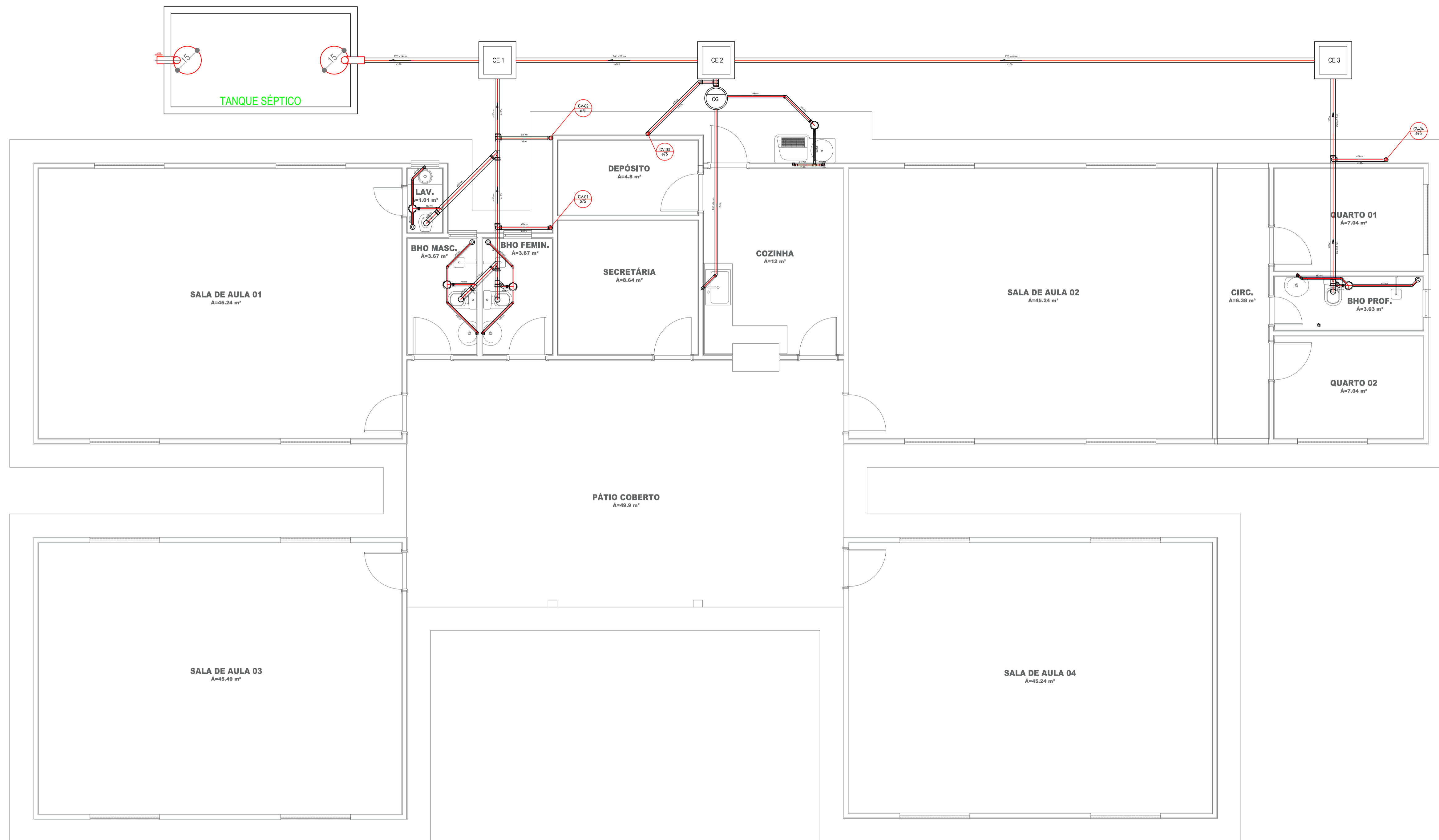
1 Planta Sanitária 1 : 50
