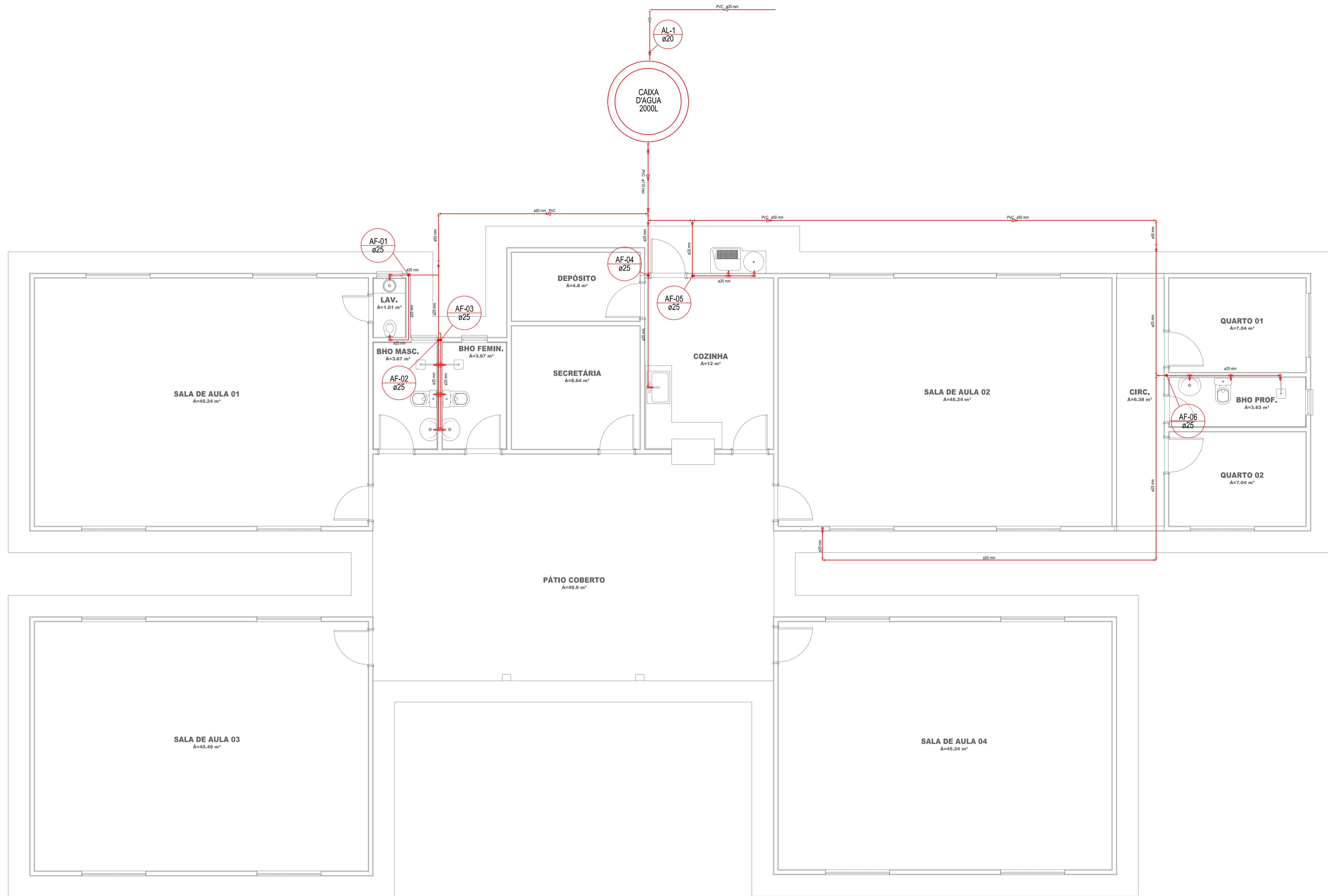
1 Planta Hidráulica 1 : 50
