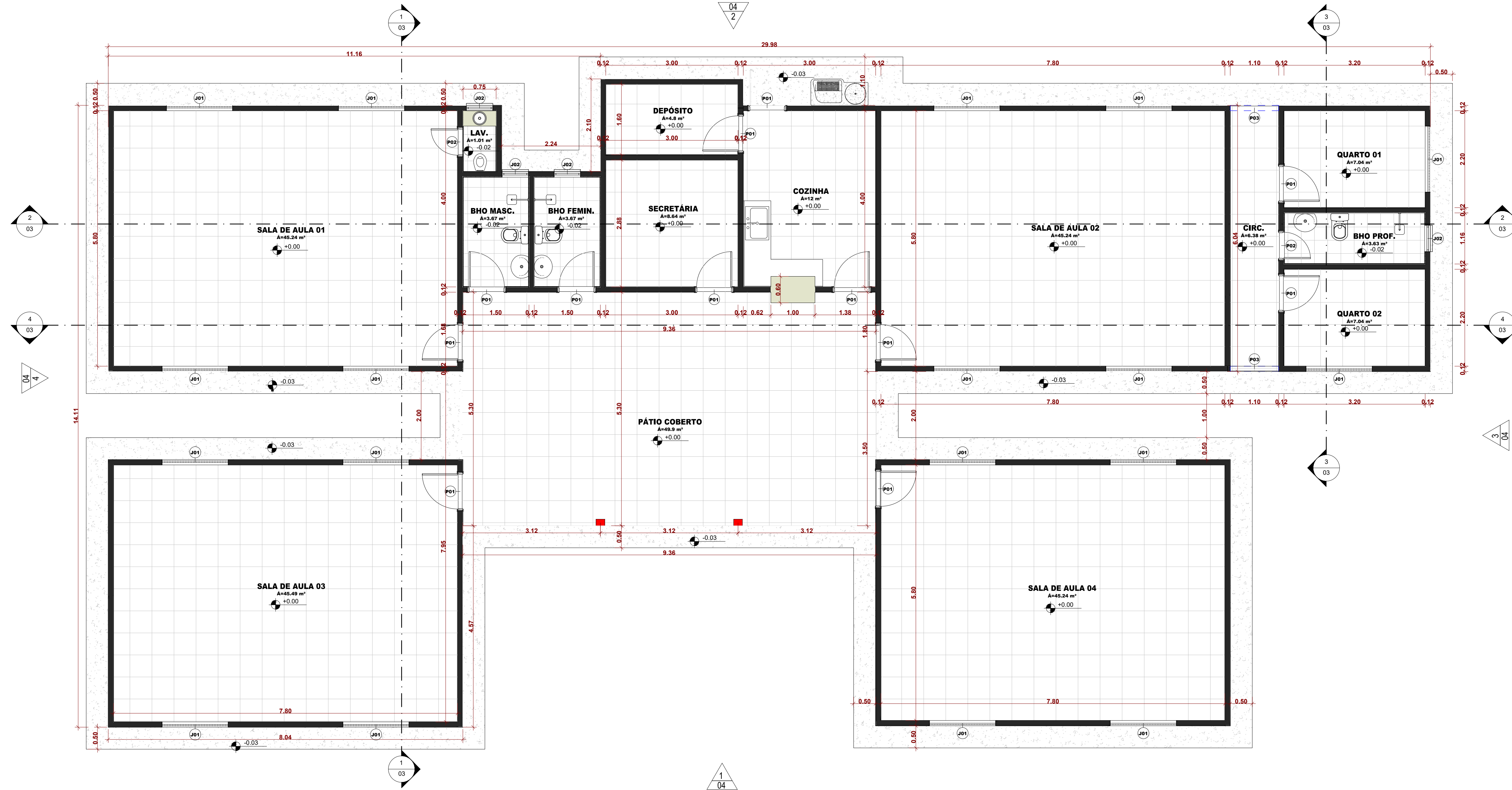
1 Planta Baixa 1:50
