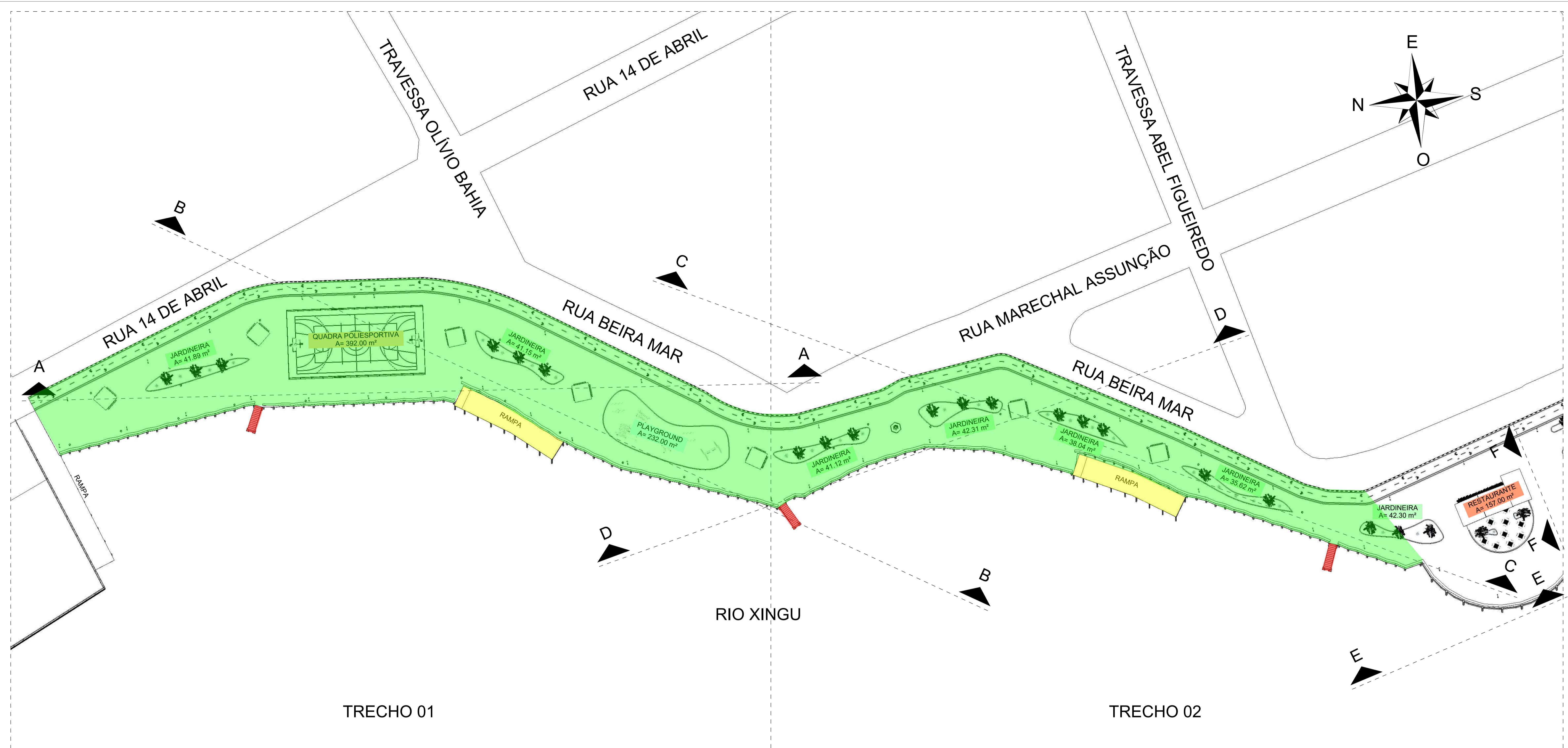
PLANTA BAIXA ESC 1:400
